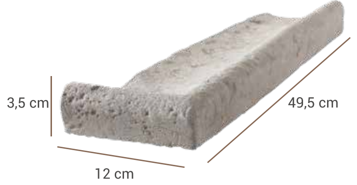
Jamb-right Jambage-droit Sağ Söve
